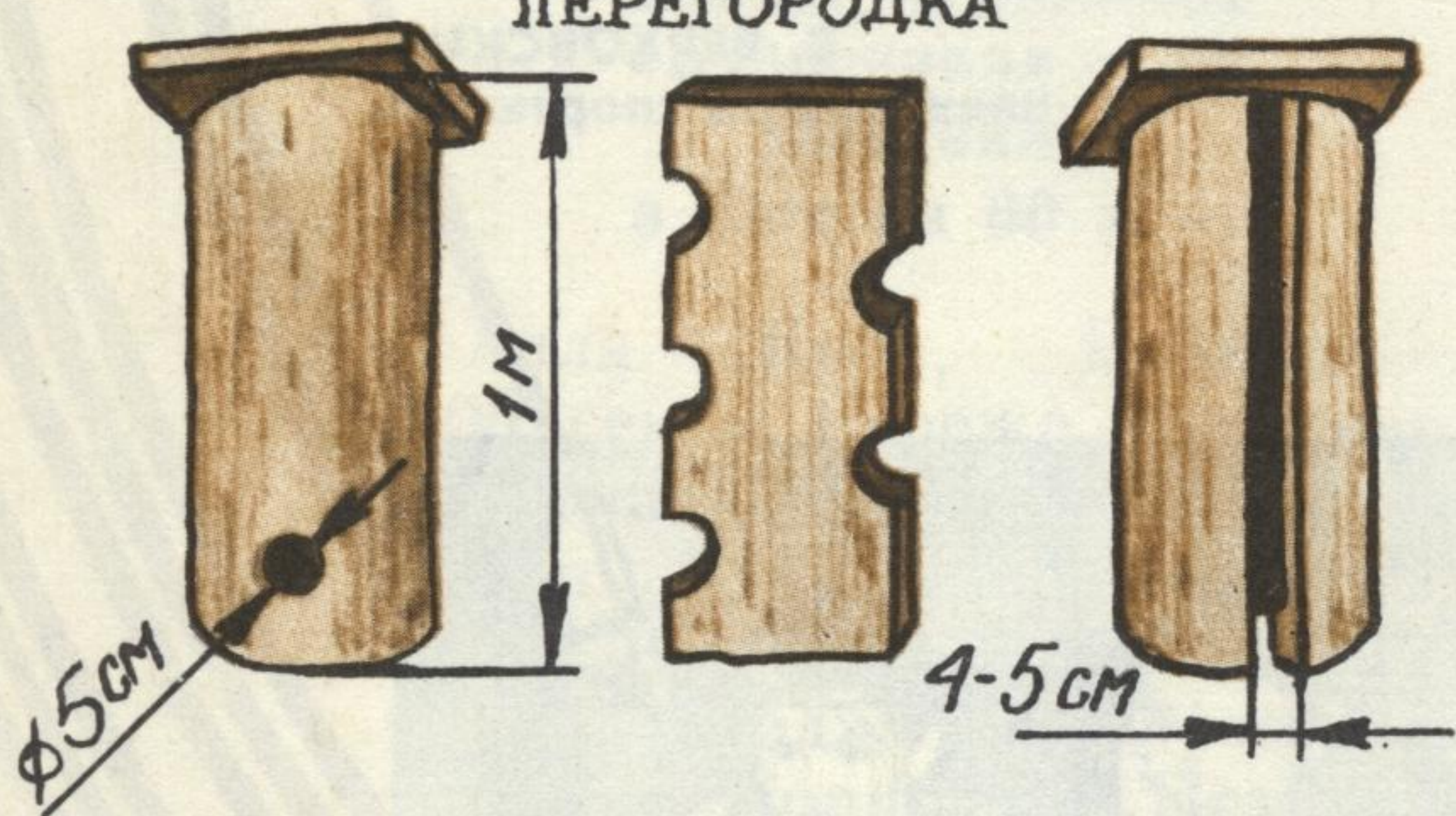
ПЕРЕГОРОДКА
